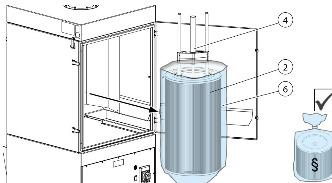
Fig. 11: Remover o cartucho filtrante
