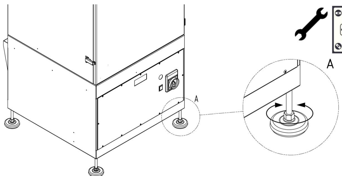
Fig. 2: Alinhar o produto
