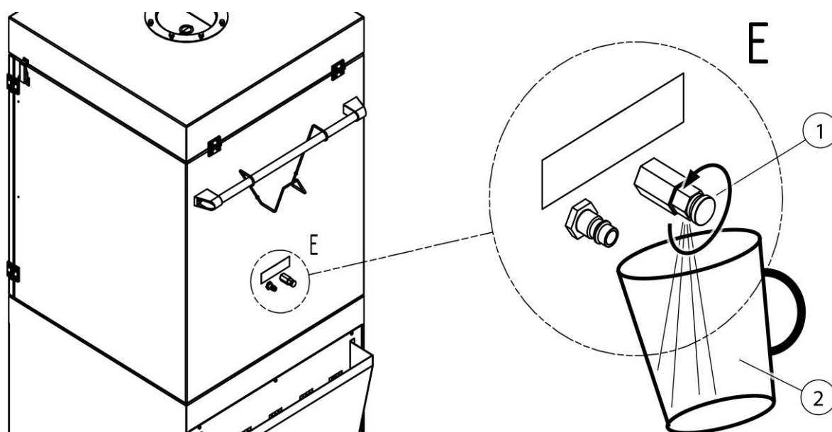
Fig. 8: Drenar o condensado
