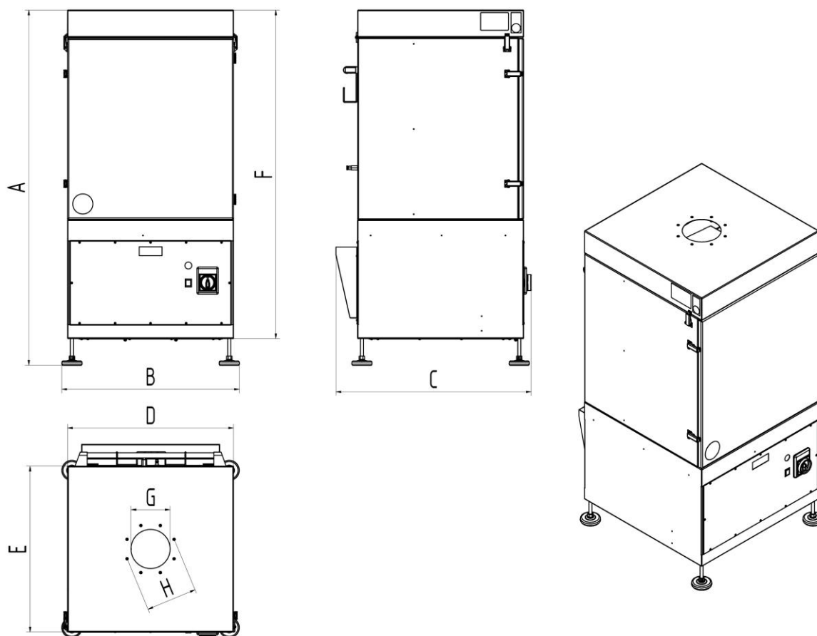
Fig. 13: Folha de dimensões
